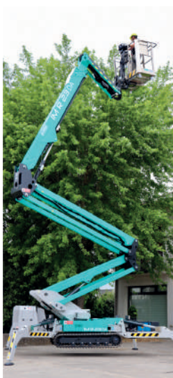
Flèche à double articulation avec section télescopique et flèche hydraulique pour assurer une excellente manœuvrabilité et un bon positionnement.
