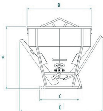
Benne conique à fond ouvrant avec goulotte latérale
